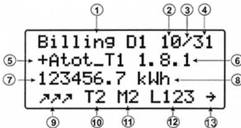
Рисунок 2-3. Информационные поля индикатора счетчика.
