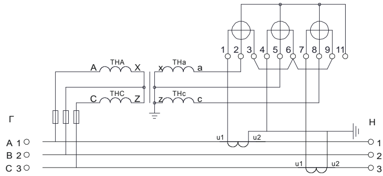
Рис. 8-2.5. С двумя измерительными трансформаторами тока и трансформаторами напряжения в фазах А и С, без нейтрали, с заземленной средней точкой.
