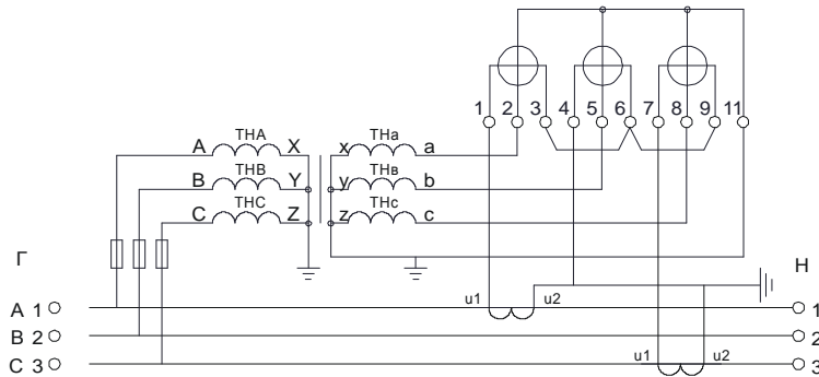
Рис. 8-2.2. С двумя измерительными трансформаторами напряжения, с заземленной нейтралью.
